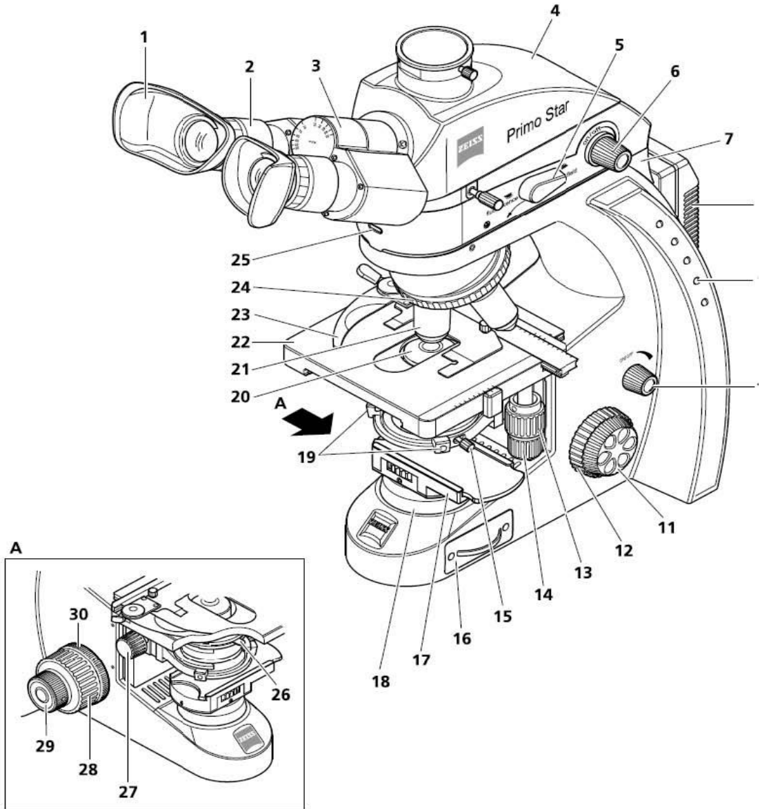
Fig. 15 Controls of Primo Star iLED
